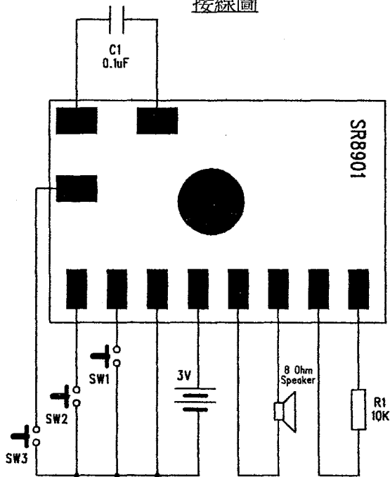
接線圖
