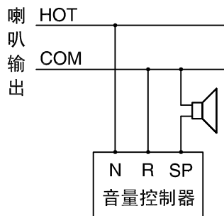
二线制连接
