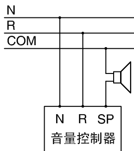
三线制连接
